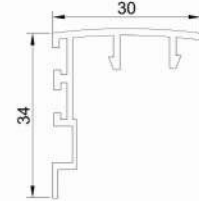
درپوش لنگه gap Code : 14321 weight : 0.33 kg/m
