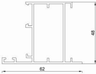
پروفیل کتیبه Engraving profile Code : 12311 weight : 0.84 kg/m
