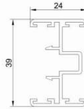
پروفیل وسط ۴ لنگه Double rickety Code : 750 weight : 0.49 kg/m
