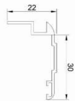
روکوب ۳۰ Suppressed the binding Code : 10023 weight : 0.23 kg/m
