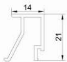
زهواردوجداره Double rickety Code : 12351 weight : 0.2 kg/m
