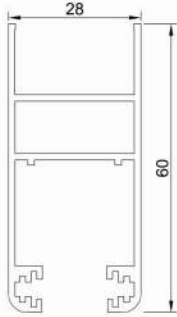
پروفیل لنگه Vent profile Code : 14331 weight : 0.8 kg/m
