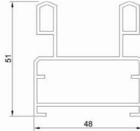
پروفیل فریم Frame profile Code : 14311 weight : 0.99 kg/m
